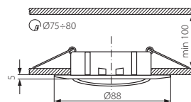
LUTO CTX-DT02B-C/M
