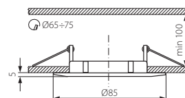
LUTO CTX-DS02B-C/M
